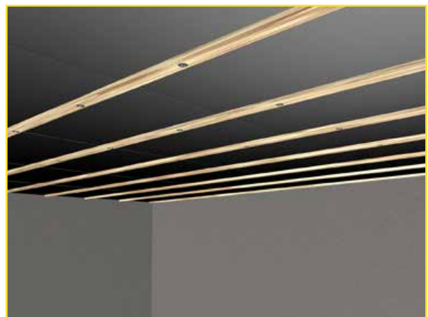
Abb.19: Fixe Befestigung der Bahnen - Entfernen der Hilfsnägel
