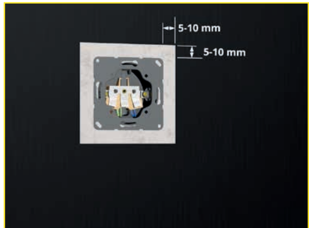
Abb.7: Halten ca. 5-10mm Sie Abstand zu Steckdosen- und Schaltereinsätzen.
