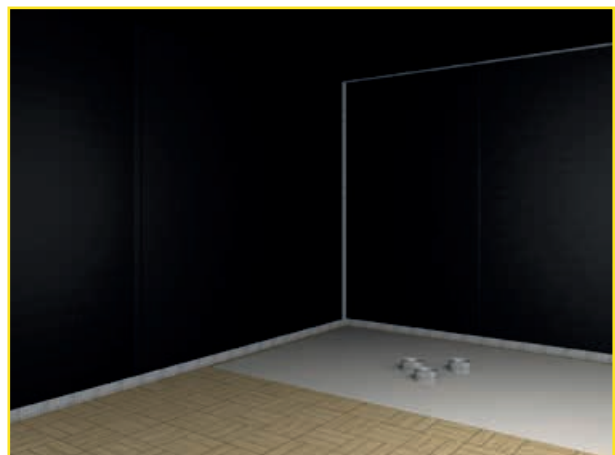
Abb.8: Aufkleben des elektrisch leitfähigen Erdungsbandes AEB im Sockelbereich. Soll der Deckenbereich geschirmt werden, wird das Erdungsband nach oben geführt und über die gesamte Deckenbreite verklebt (Immer gegen die Verlegerichtung).
