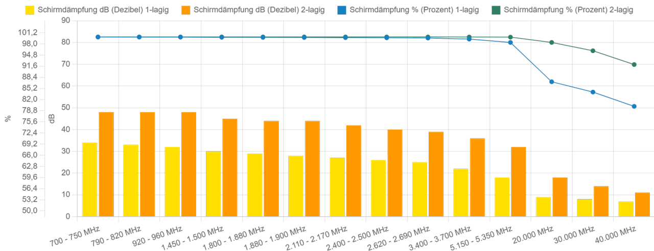
Schirmdämpfung - Topas+ - 700 MHz bis 40.000 MHz (40 GHz)
